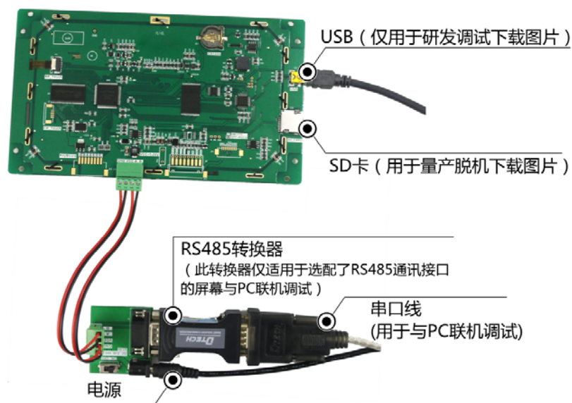
图 1-5 调试工具图
