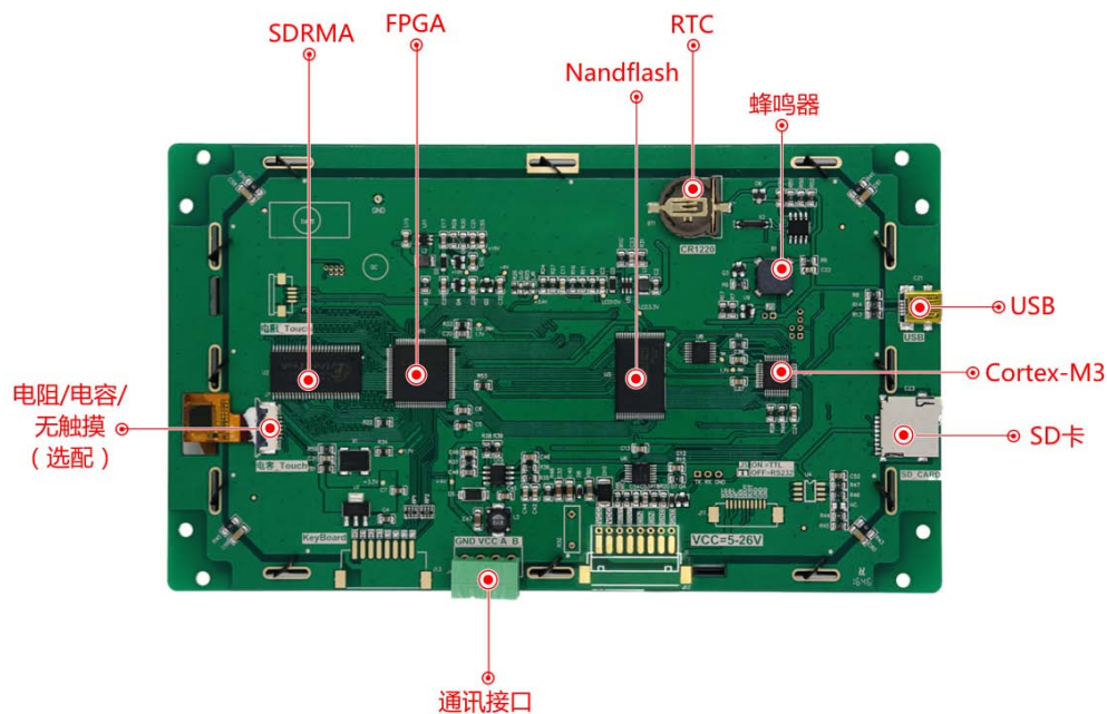
图 1-4 硬件配置图
